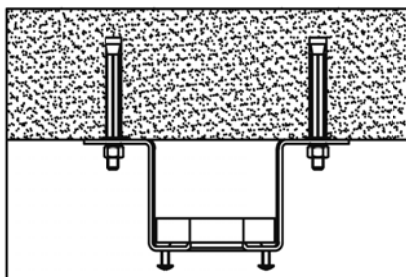
SOPORTE MONTAJE
